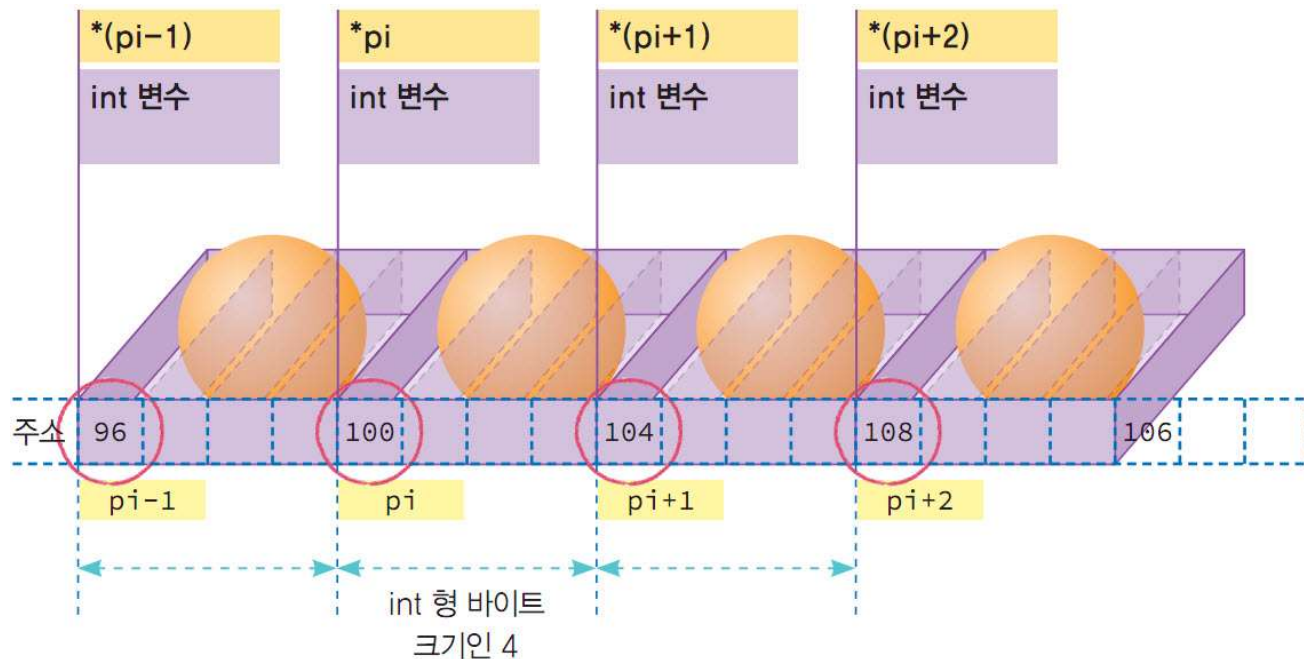
그림 8-10 주소의 연산을 이용한 이웃한 변수의 참조
