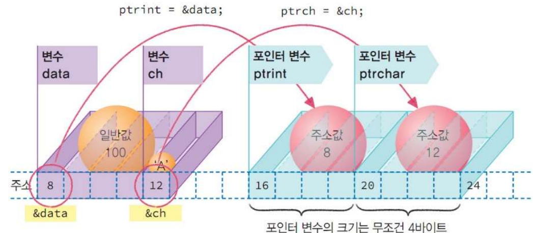
그림 8-9 포인터 변수와 주소값이 저장된 변수 사이의 관계
