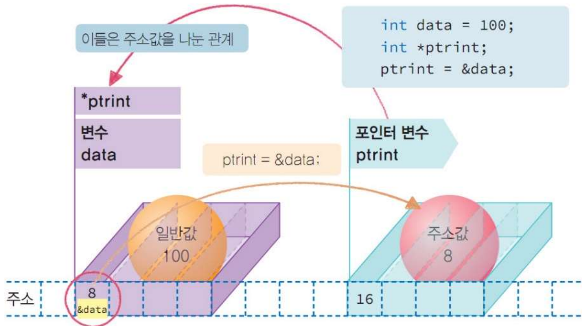
그림 8-6 포인터 변수선언과 주소의 대입
