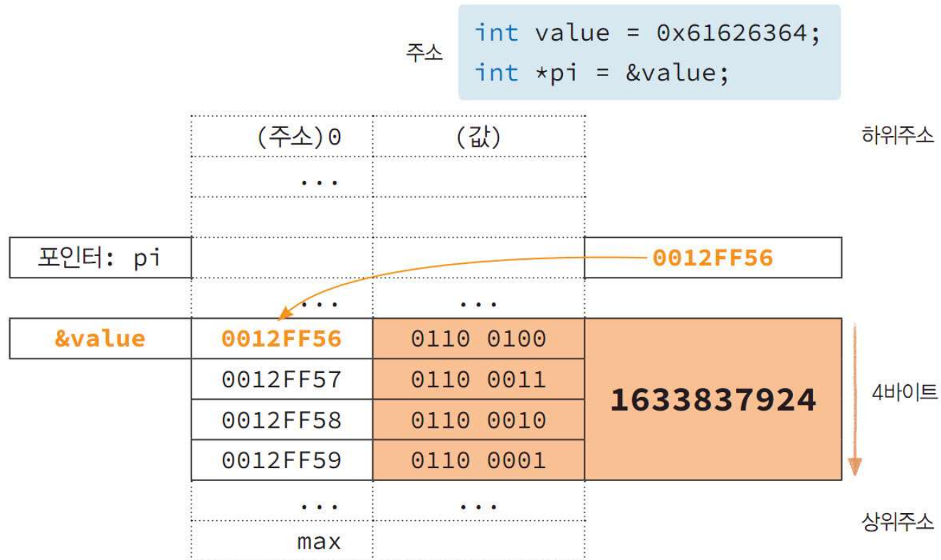
그림 8-12 지역변수가 선언된 메모리 내부 모습
