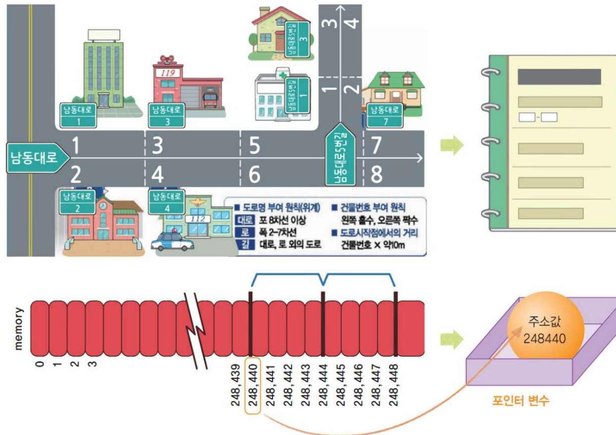
그림 8-3 메모리 주소를 저장하는 포인터 변수
