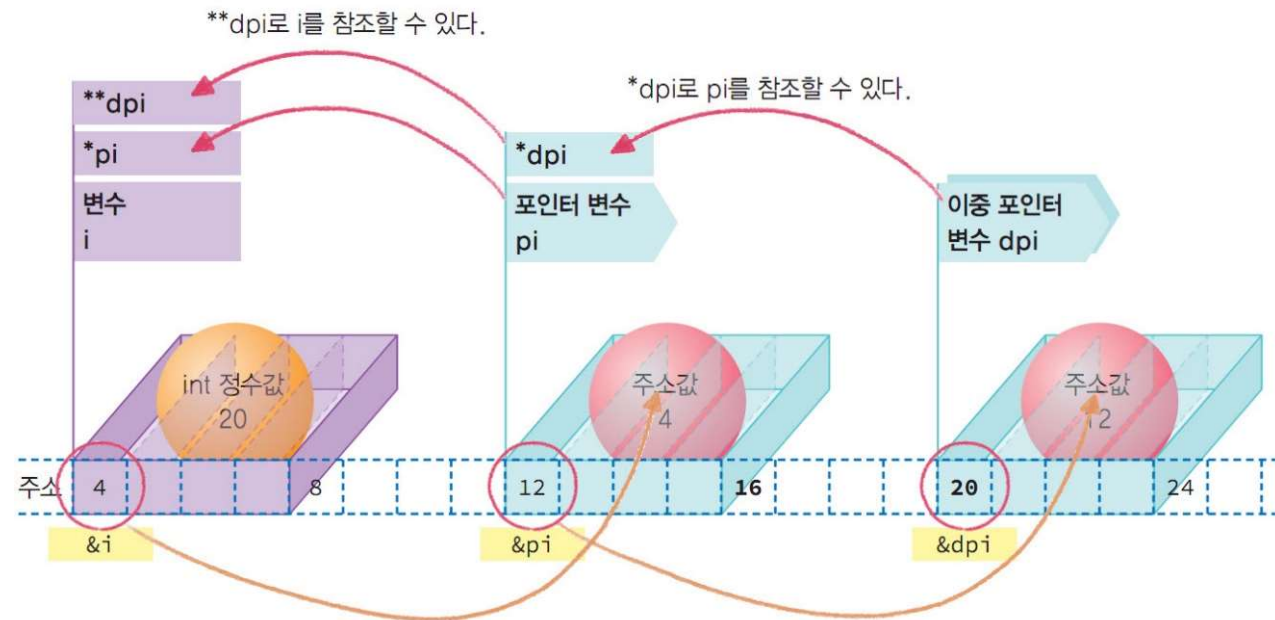
그림 8-15 이중포인터의 메모리와 변수
