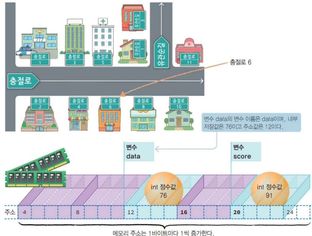
그림 8-1 메모리 주소
