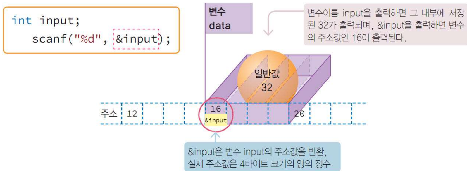
그림 8-2 주소연산자 & 이해
