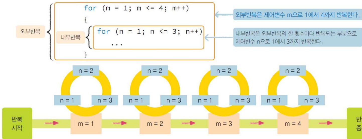
그림 7-33 중첩된 for문에서 제어변수의 변화(외부반복 제어변수: m, 내부반복 제어변수: n)
