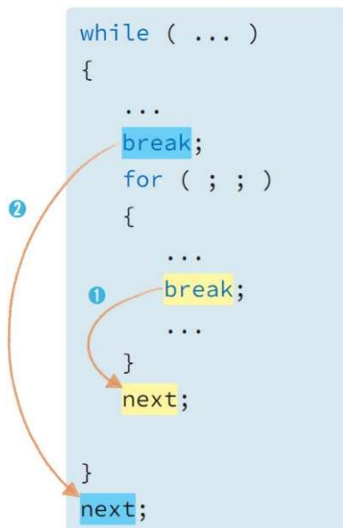
그림 7-28 중첩된 반복문의 break
