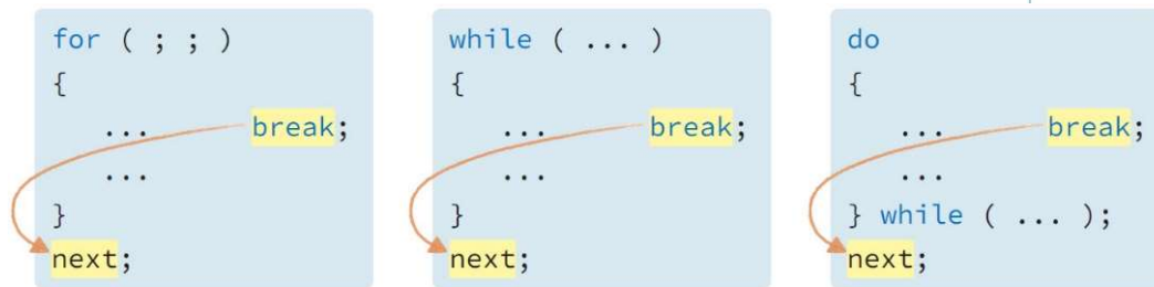
그림 7-27 반복문의 break
