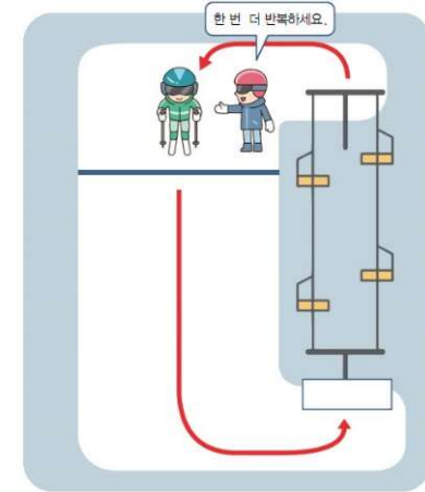
그림 7-2 while 반복
