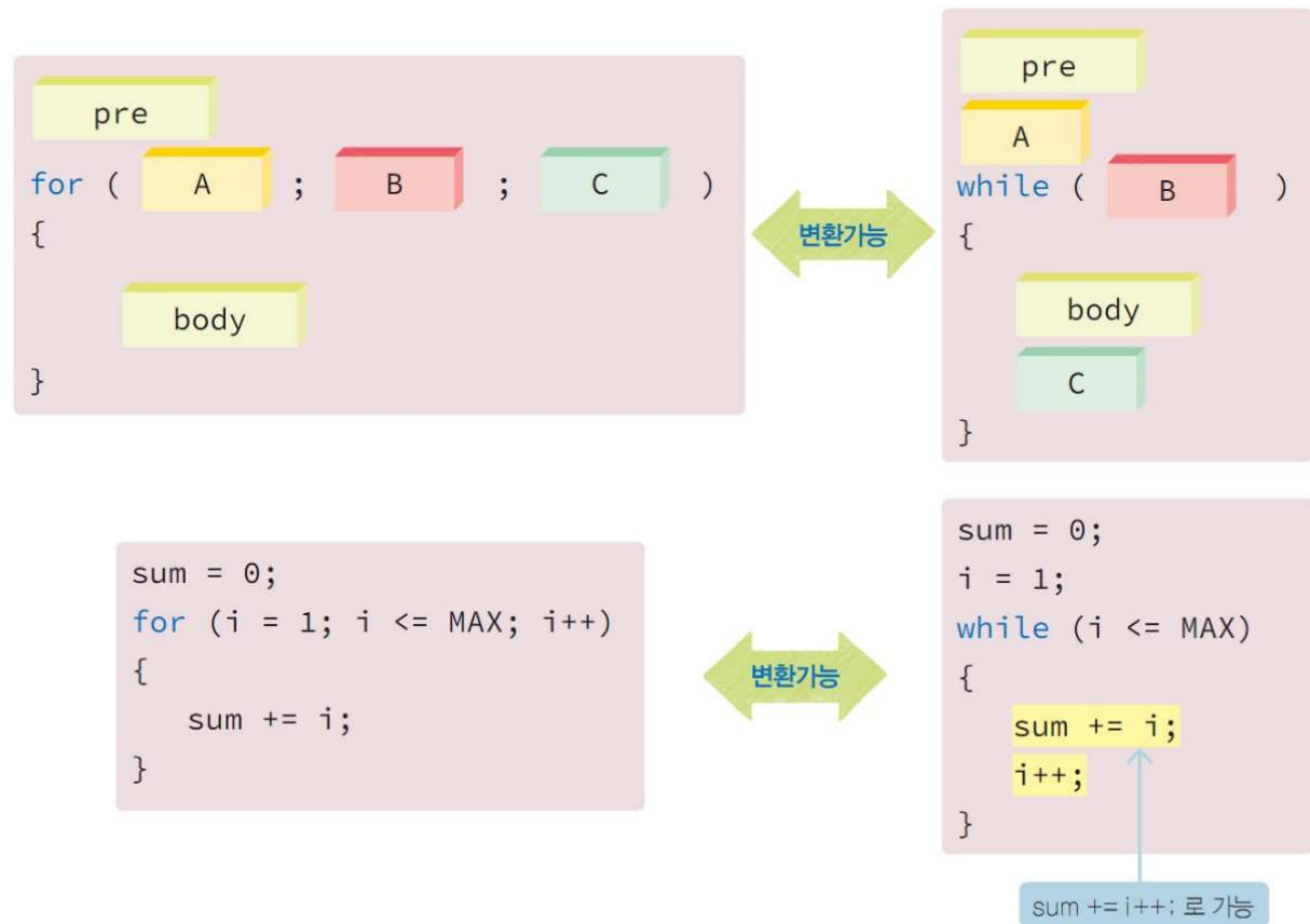
그림 7-25 반복문 for와 while간의 변환
