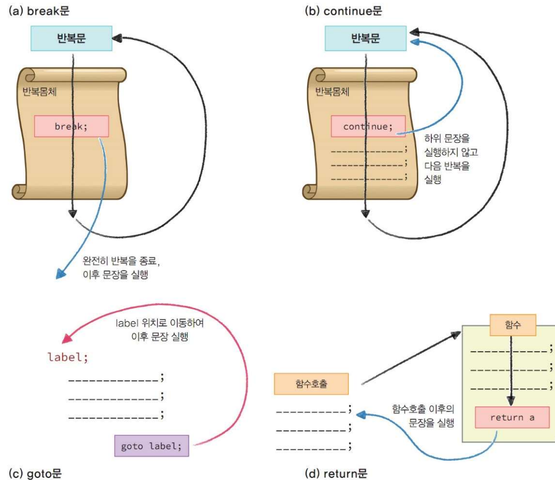
그림 7-26 여러 분기문의 개념
