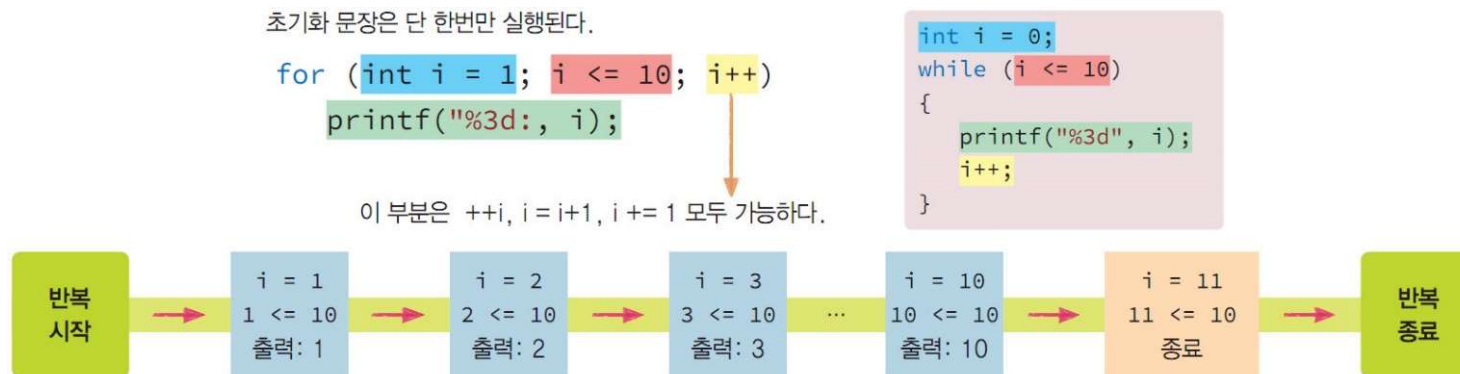
그림 7-17 1부터 10까지 출력하는 for문
