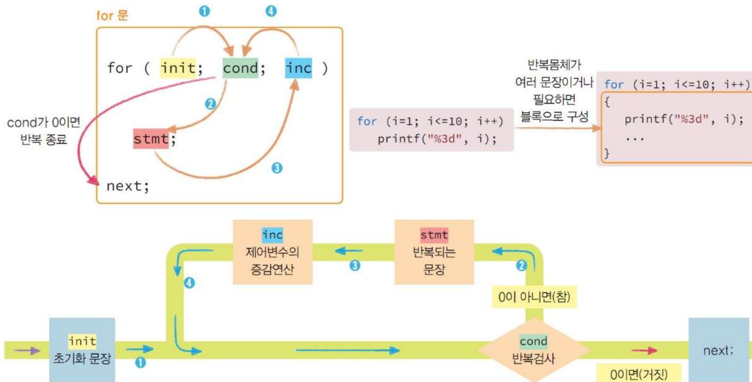
그림 7-16 반복 for문의 제어흐름
