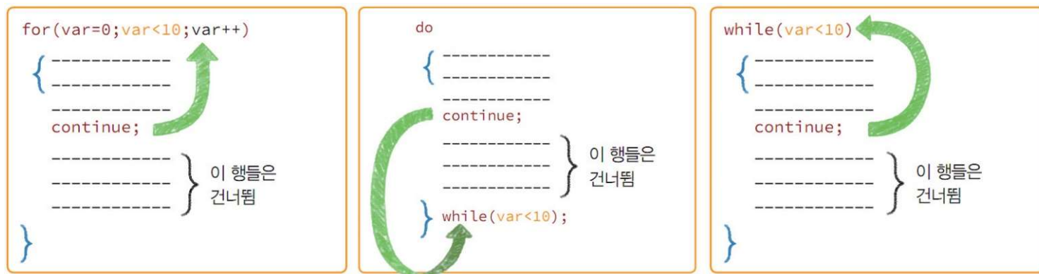
그림 7-29 다양한 continue문 이후의 실행 순서
