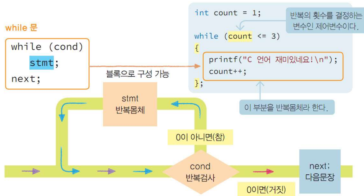
그림 7-9 반복 while문과 제어흐름
