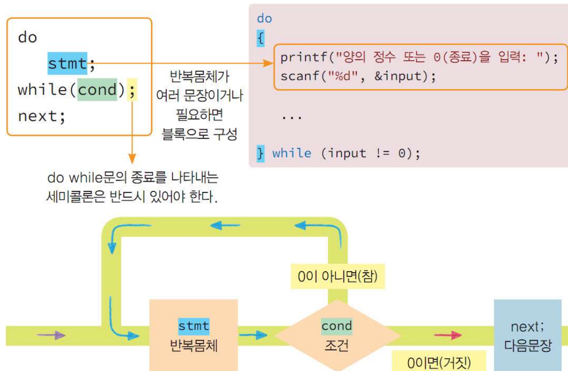
그림 7-14 반복 do while문의 제어흐름
