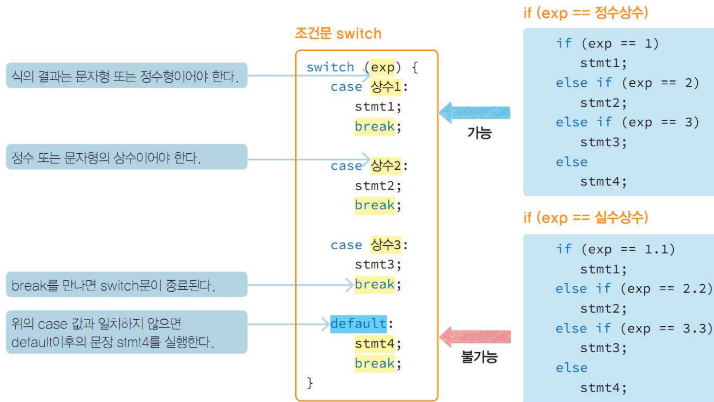
그림 6-19 switch 문 문장구조
