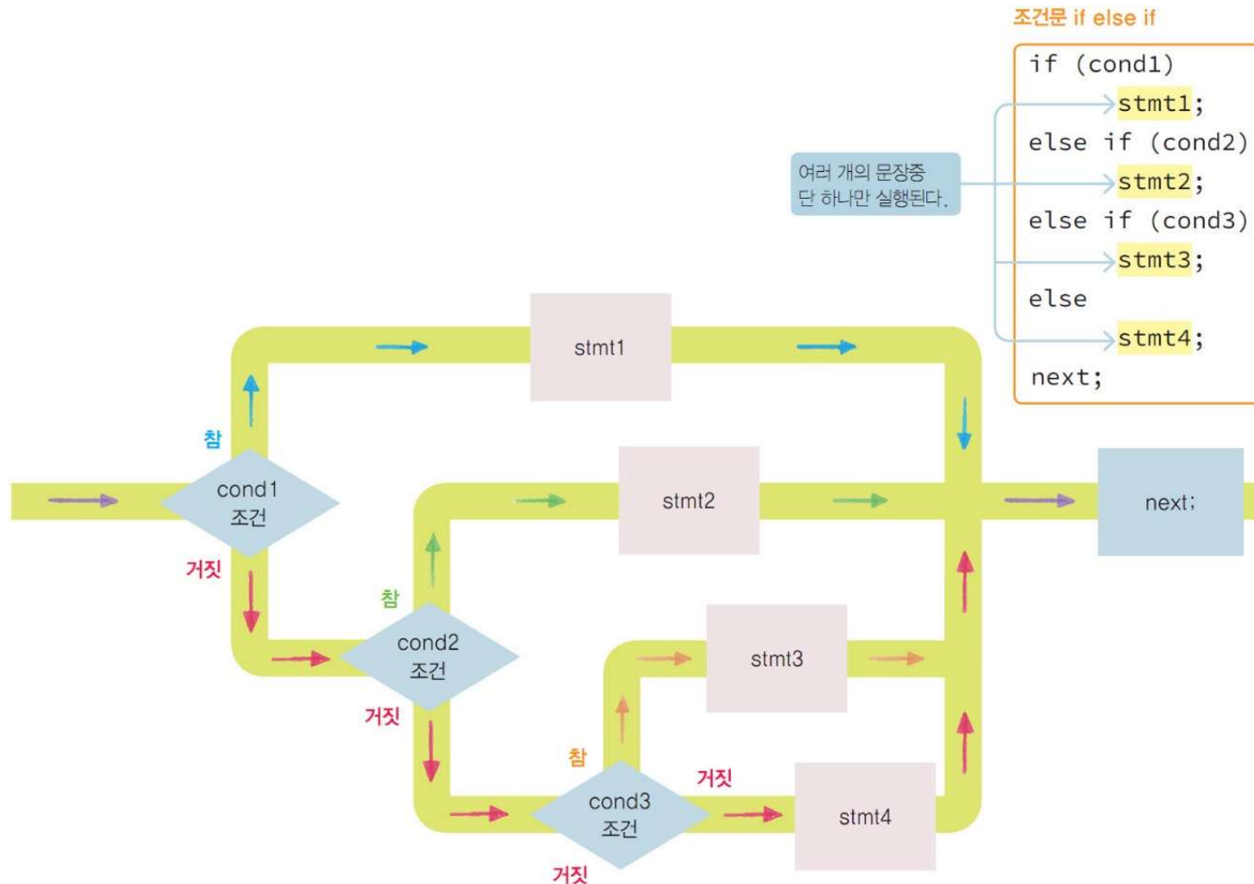
그림 6-13 조건문 if else if 문의 제어흐름
