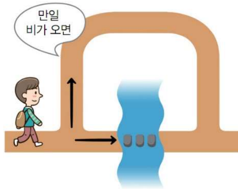
그림 6-6 길의 선택
