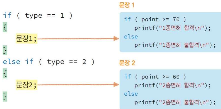
그림 6-15 중첩된 if
