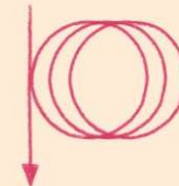
그림 6-3 반복순환
