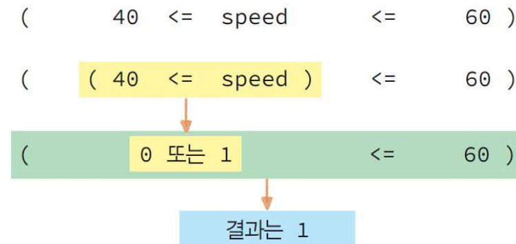
그림 6-18 주의해야 할 조건 연산식
