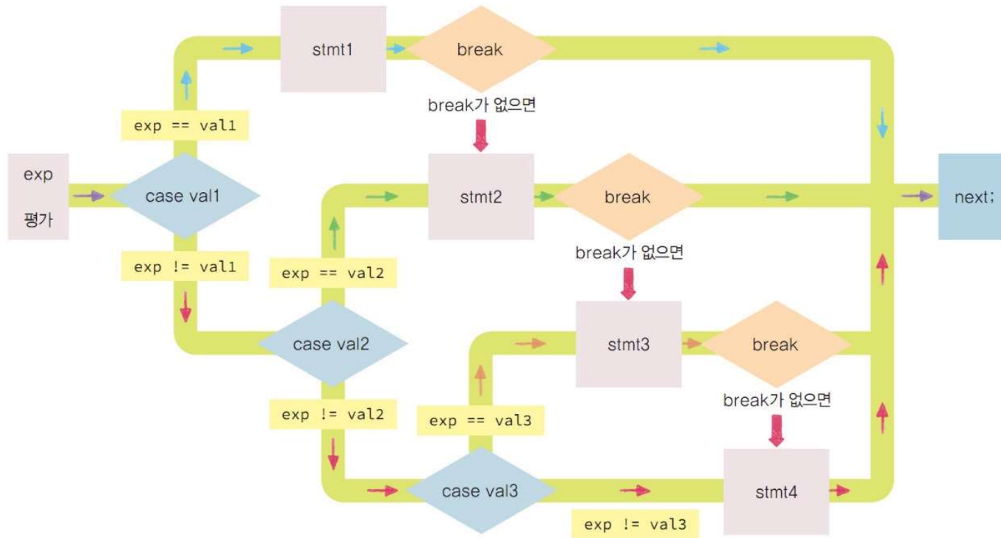
그림 6-20 switch 문의 제어흐름
