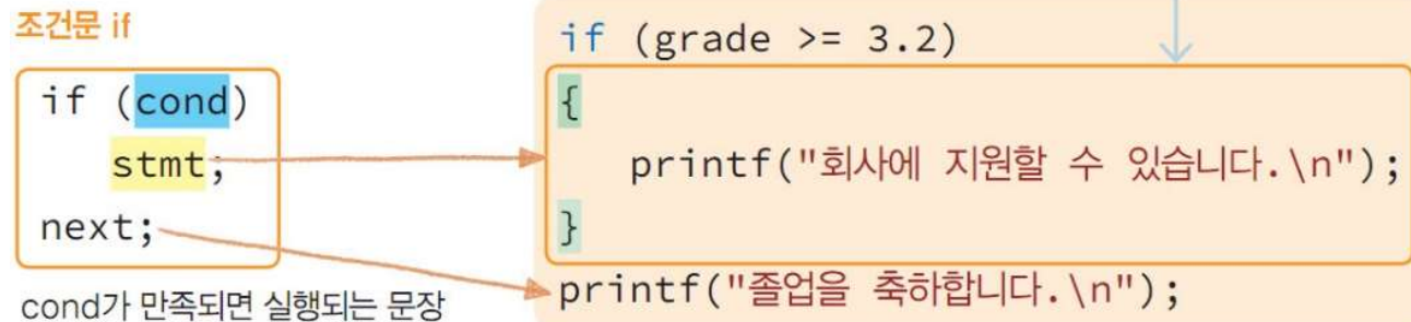
그림 6-8 if 문
